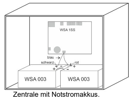
Zentrale mit Notstromakkus.
