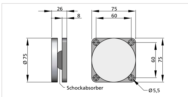
Standardanker ASV 75
