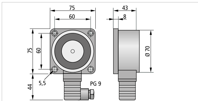
Haftmagnet THM 443
