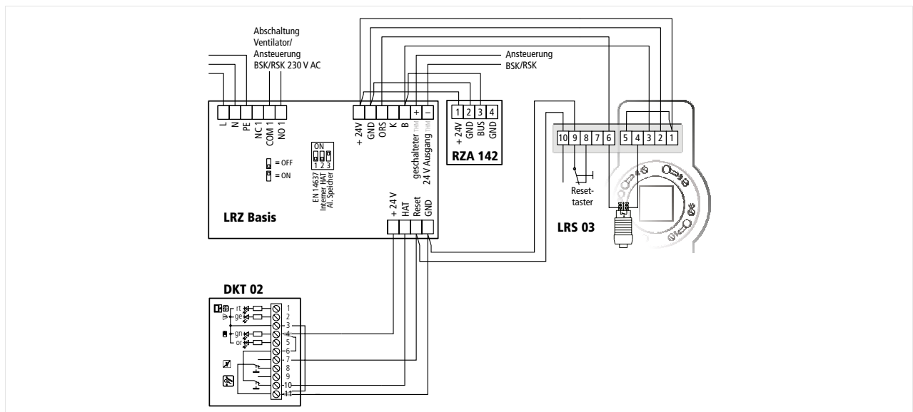
Abb. 8: Anschlussbeispiel LRS 03 mit LRZ Basis und DKT 02
