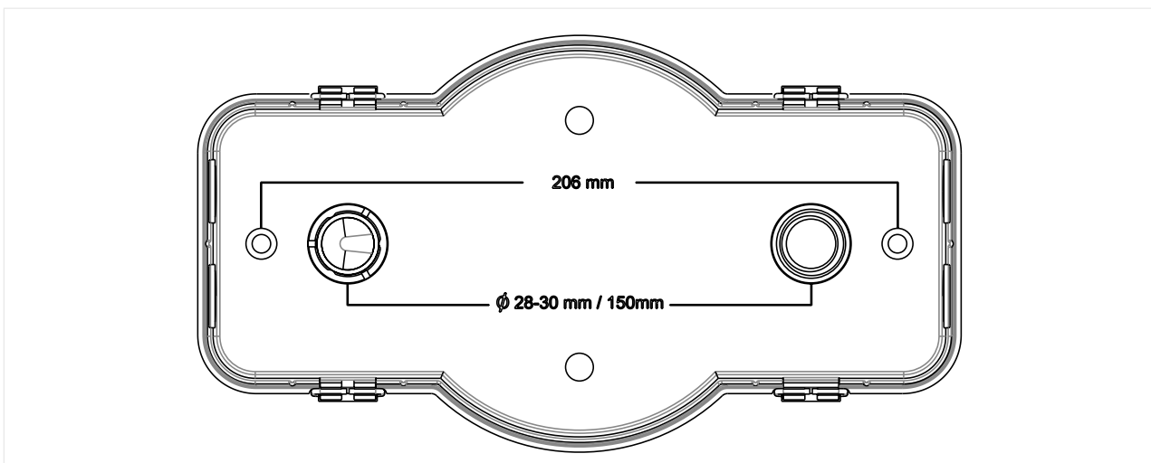
Abb. 5: Bohrmaße
