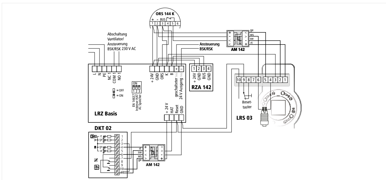
Abb. 11: Anschlussbeispiel LRS 03 mit LRZ Basis, ORS 144 K und DKT 02 (mit Leitungsüberwachung)
