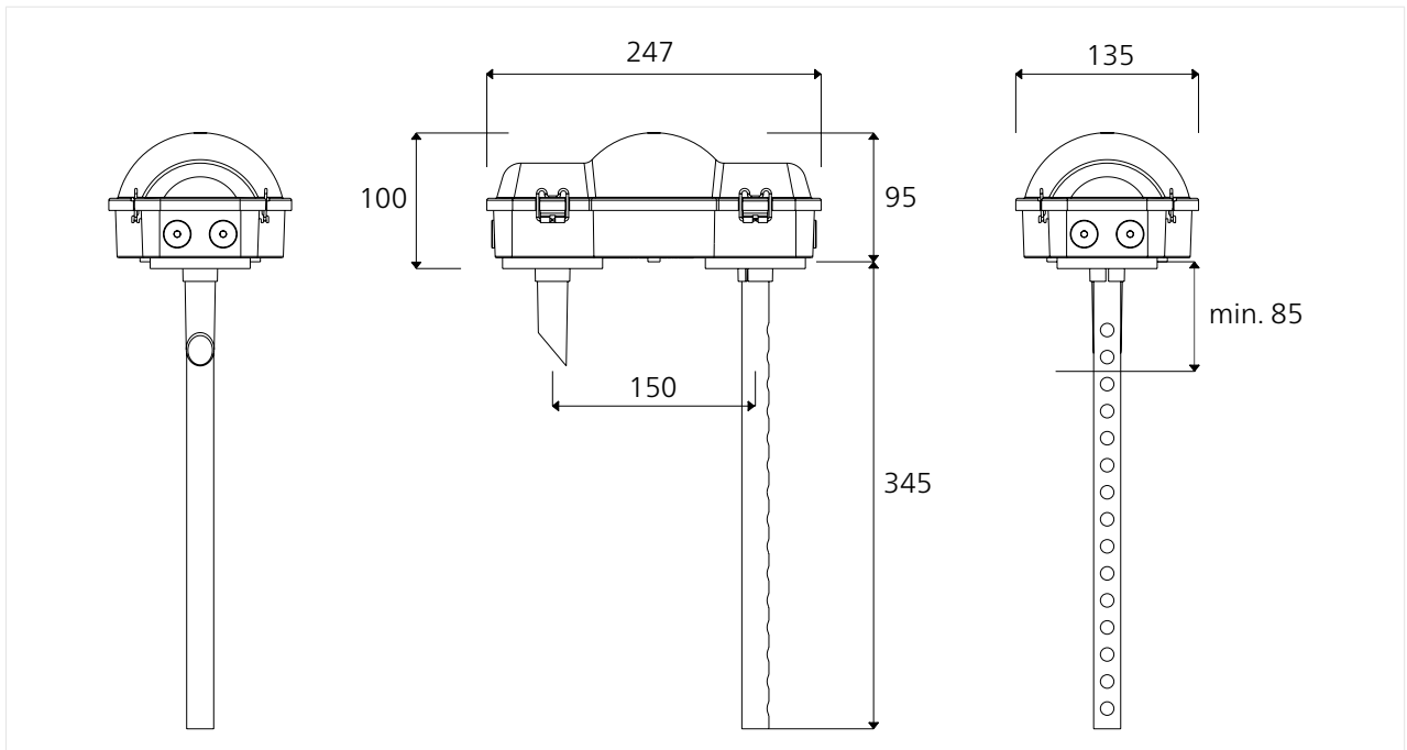
Abb. 3: Maßbild
