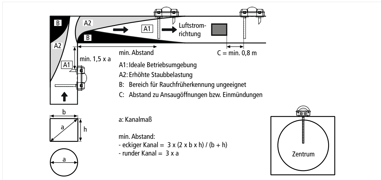
Abb. 2: Projektierungsübersicht
