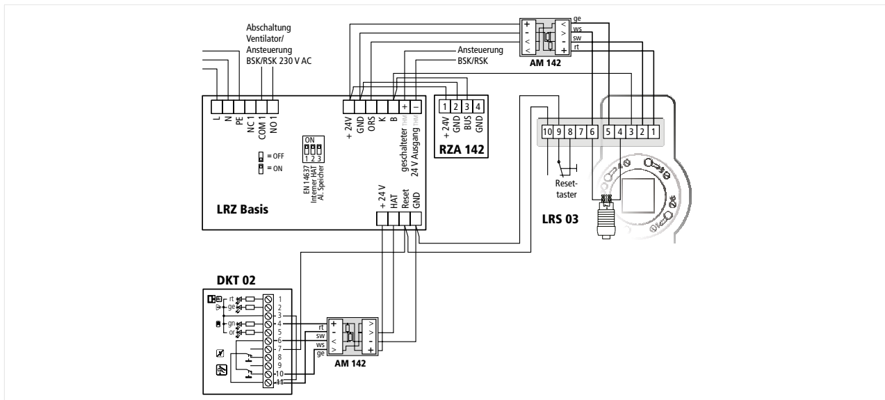
Abb. 10: Anschlussbeispiel LRS 03 mit LRZ Basis und DKT 02 (mit Leitungsüberwachung)
