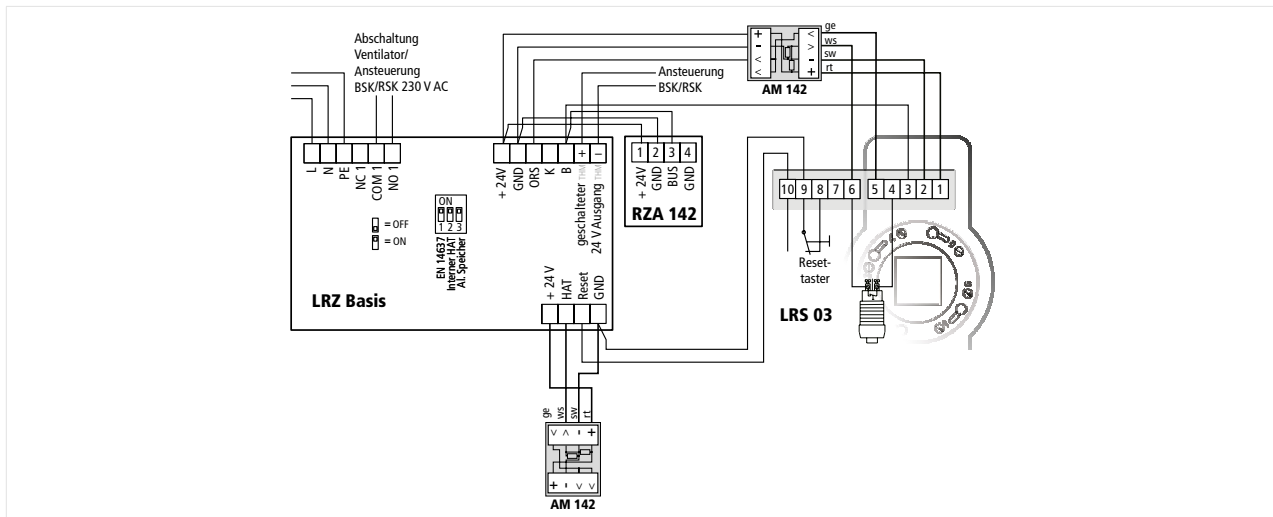
Abb. 9: Anschlussbeispiel LRS 03 mit LRZ Basis (mit Leitungsüberwachung)
