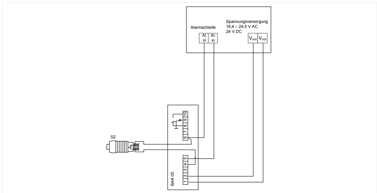
Abb. 7: LRS 03 mit AC oder DC Spannungsversorgung
