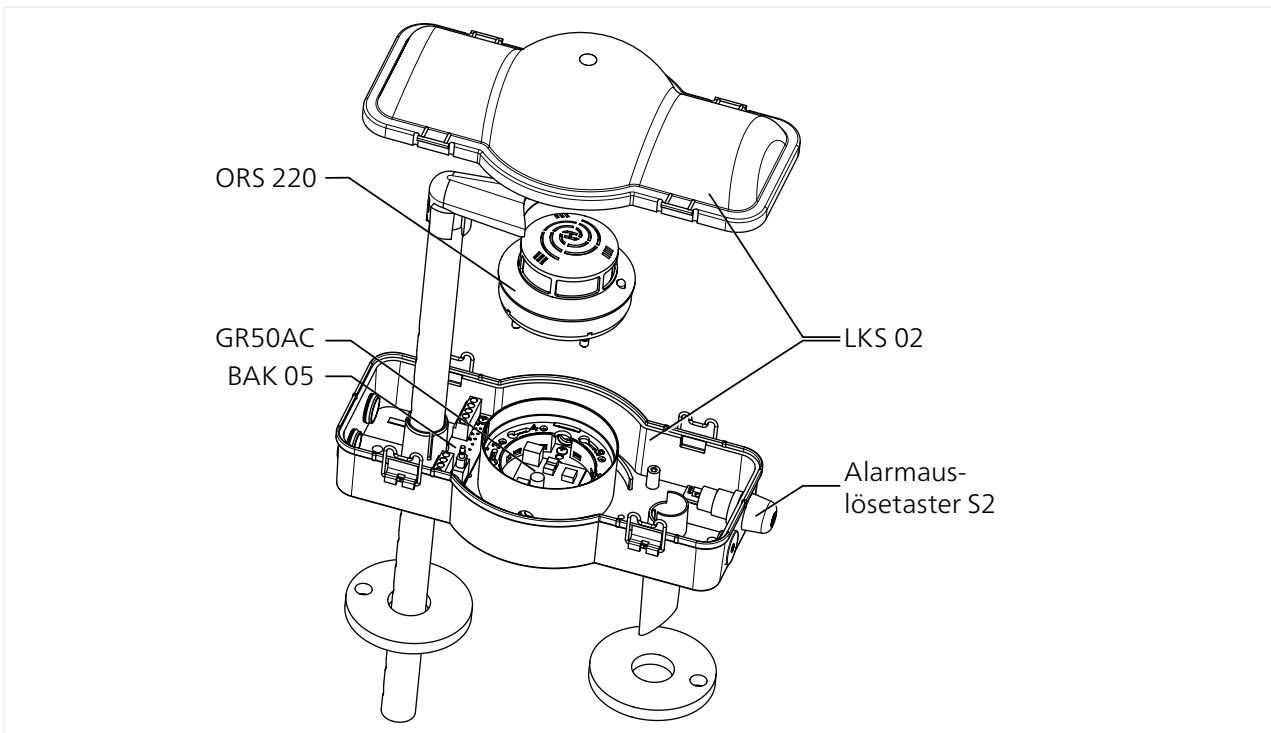
Abb. 1: Lüftungs-Rauchscharter-System LRS 03
